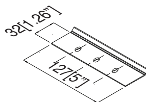
Clip de fijación muro Para espesores de panel mayores a 1.5"
